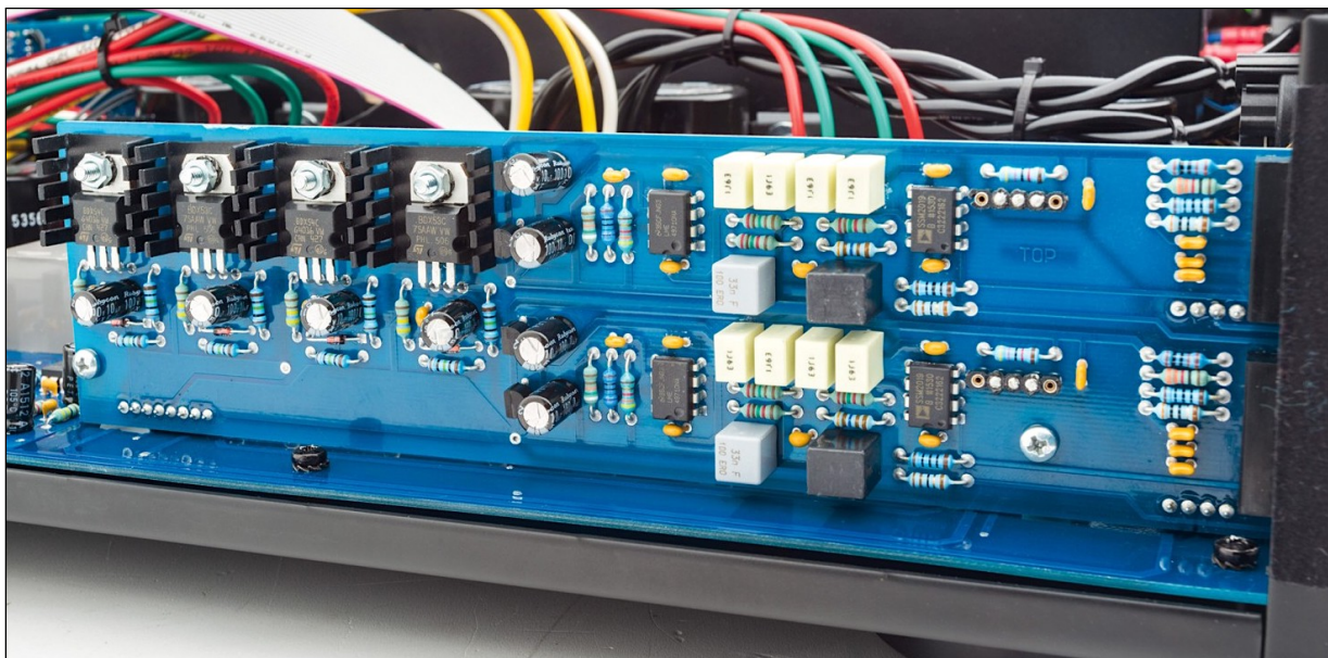
Carte phono MM/MC du modèle testé et accès par la trappe au réglage de l'impédance de charge
